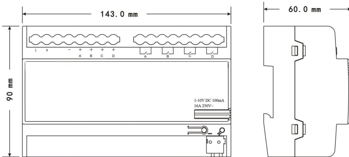
尺寸图:
