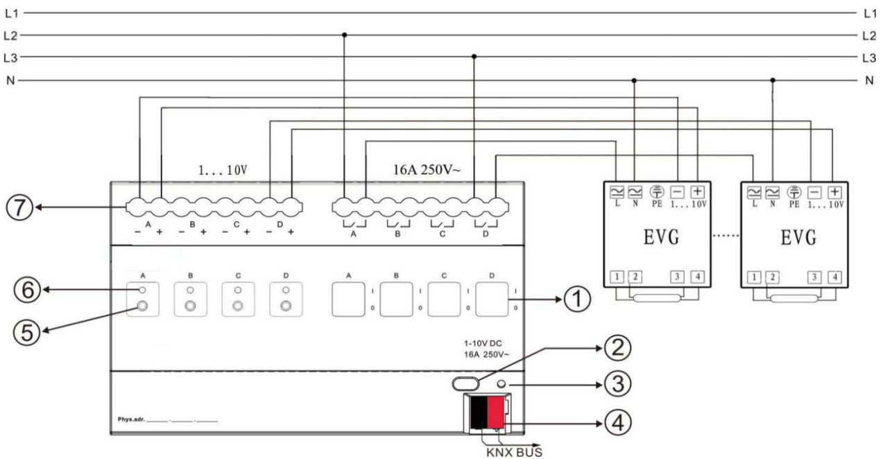
接线图:
