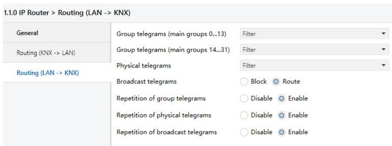
图 5.3 “Routing(LAN->KNX)”参数设置界面
