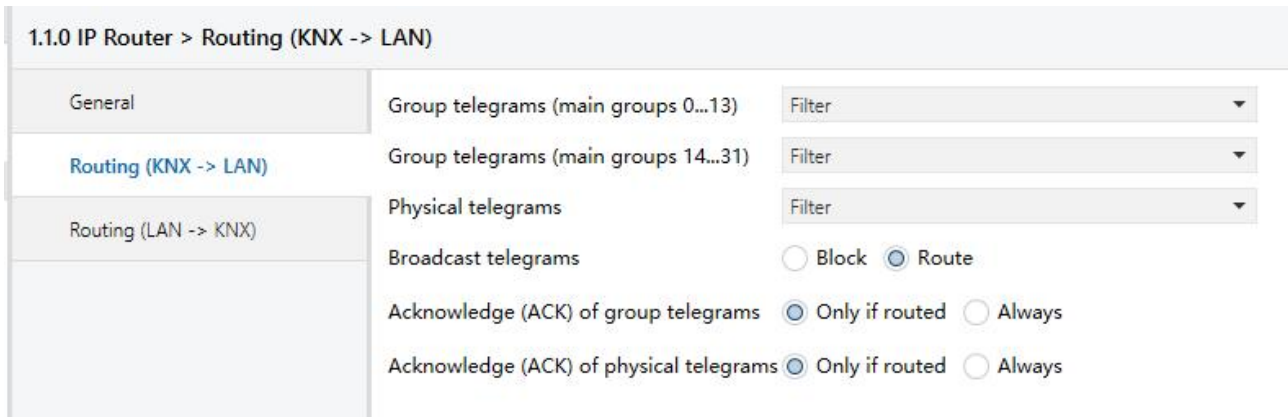
图 5.2 “Routing(KNX->LAN)”参数设置界面
