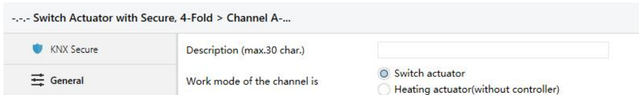
图 4.3 “Channel X”参数设置界面
