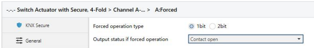
图 4.4.7 X: Forced 设置界面
