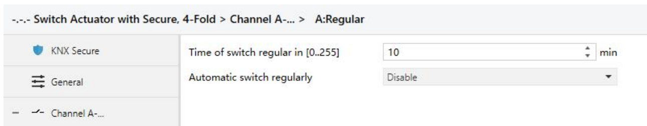
图 4.5.3 X: Regular 参数设置界面
