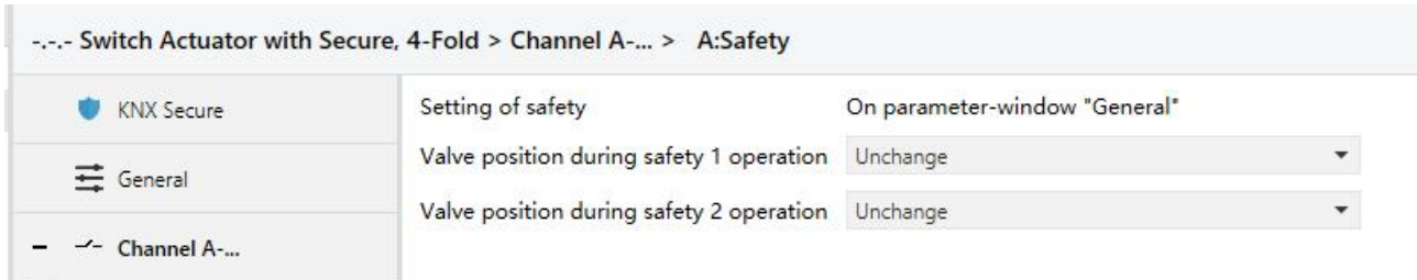
图 4.5.4 X: Safety 参数设置界面
