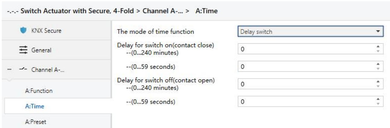
图 4.4.1.1 X: Time-Delay
