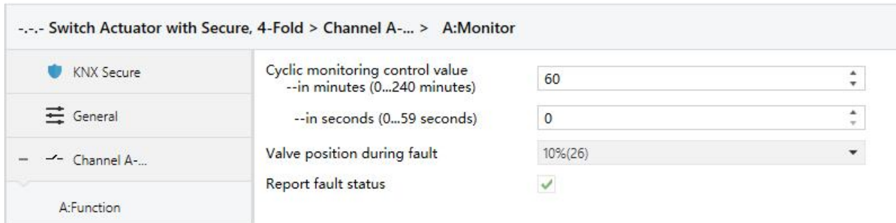
图 4.5.1 X: Monitoring 设置界面
