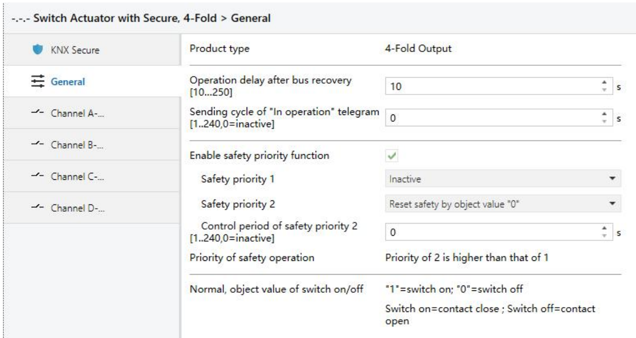
图 4.2 “General”参数设置界面
