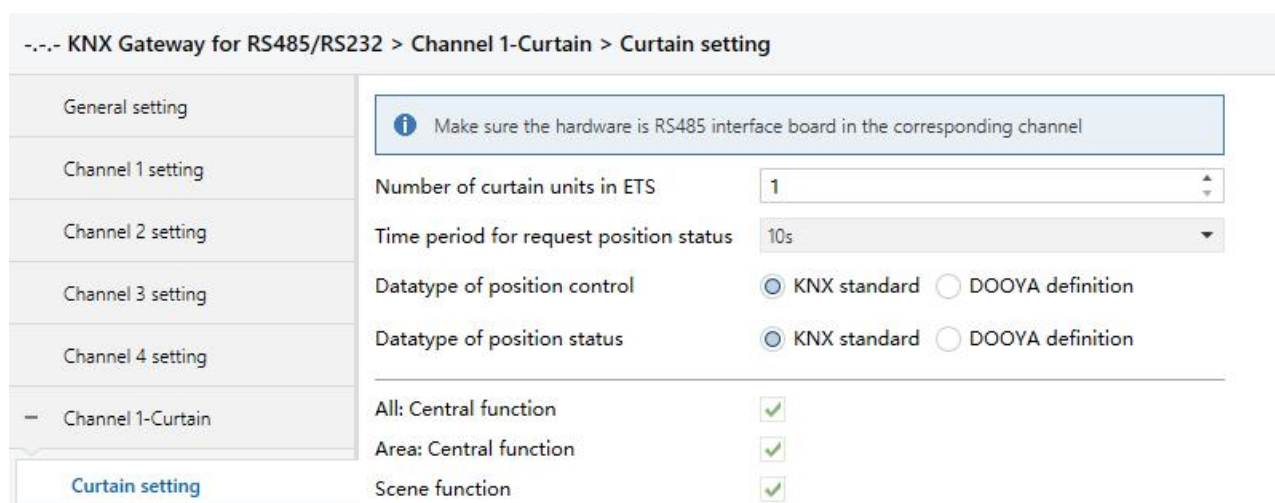
图 5.6.1 “Curtain gateway” 参数设置界面
